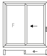
2 vie - 1 ante+fisso 2 rail-1 sash+fixed
