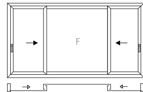
2 vie - 2 ante+fisso 2 rail-2 sash+fixed
